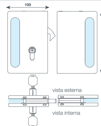
“D” APERTURA INVERSA serratura con chiave esterna/interna apertura centrale
