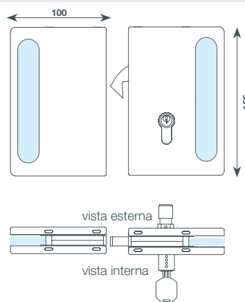
“C” APERTURA INVERSA serratura con chiave interna maniglia esterna, apertura centrale, vista interna
