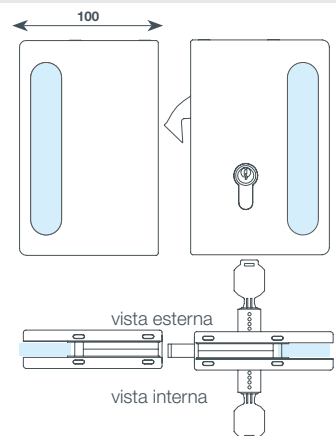
“D” APERTURA DI SERIE serratura con chiave esterna/interna apertura centrale
